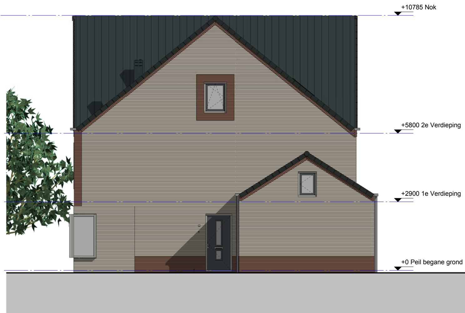
rechtergevel
