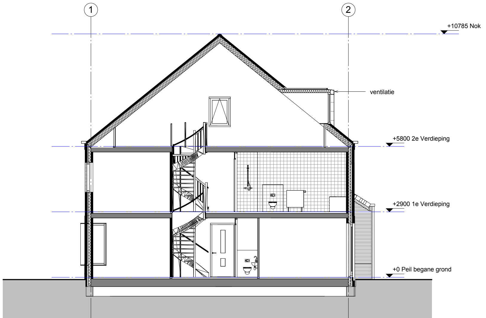
Doorsnede A132-136
