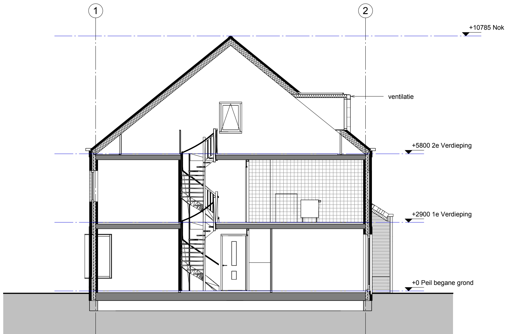
Doorsnede A-135
