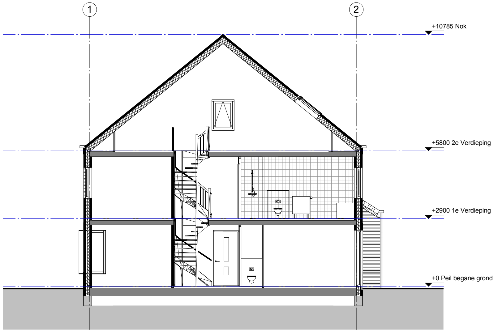
Doorsnede A132-136
